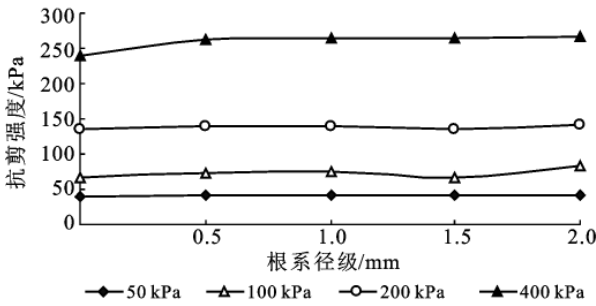
图 2 垂直布根 2 根后根土复合体抗剪强度
