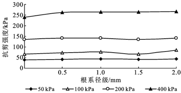
图 3 垂直水平各布 2 根后根土复合体抗剪强度
