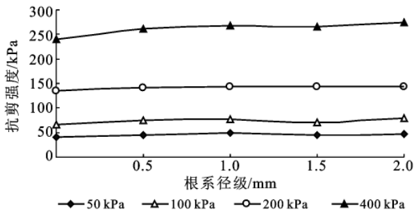
图 1 垂直布根 4 根后根土复合体抗剪强度
