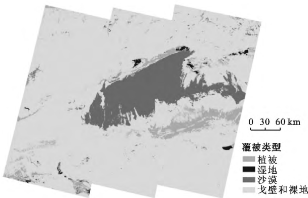
图 2 研究区 2000 年地表覆被分类图
