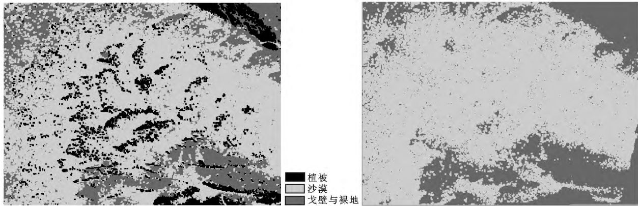
图 4 研究区沙漠转变为植被对比图
