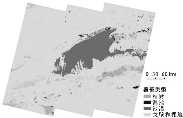
图 1 研究区 1990 年地表覆被分类图
