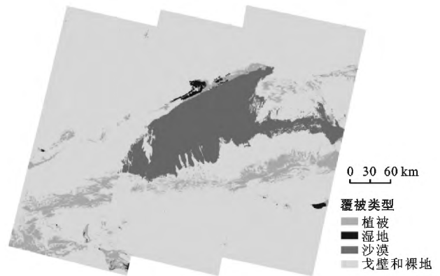
图 3 研究区 2010 年地表覆被分类图
