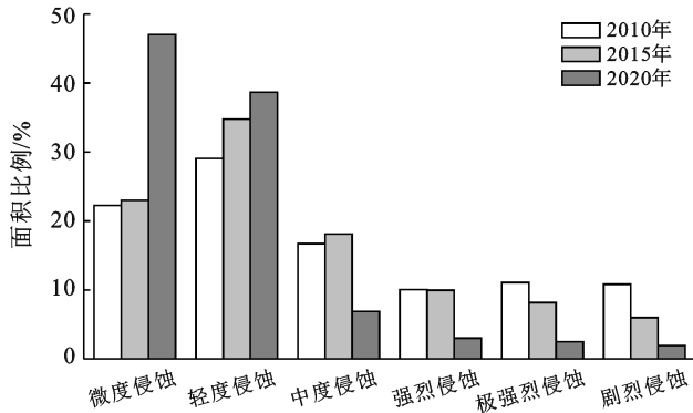
图 1 丹江口库区 2010, 2015 和 2020 年土壤侵蚀强度各等级面积比例
