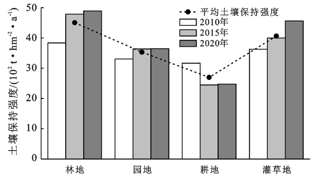
图 2 丹江口库区 2010, 2015 和 2020 年不同土地利用类型土壤保持能力统计
