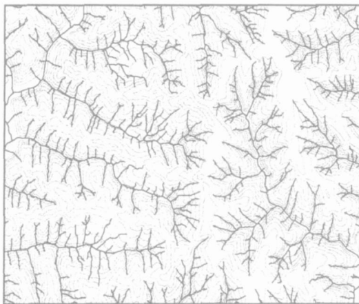
a 实际地形的沟谷网络
