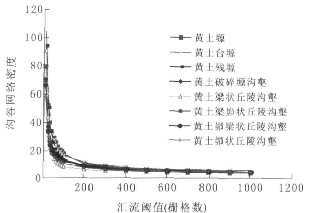
图 3 沟谷网络密度和阈值关系曲线图
