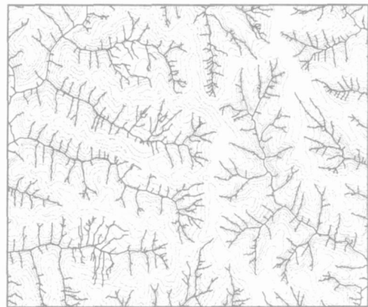
b 利用理论阈值获得的沟谷网络
