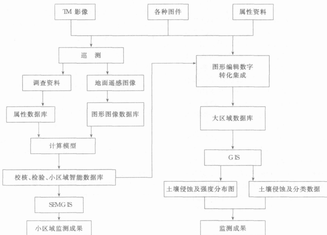
图 1 地面遥感监测系统工作流程图
