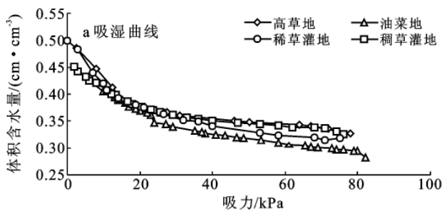
图 2 不同植被类型土壤的脱湿和吸湿过程的持水曲线
