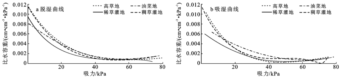
图 3 不同植被类型土壤的脱湿和吸湿时的比水容量曲线
