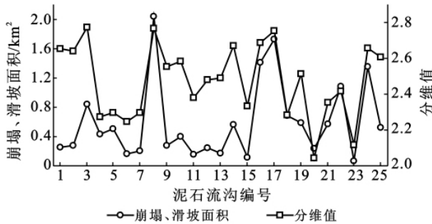
图1 泥石流堆积物分维值与崩塌、滑坡面积的关系
