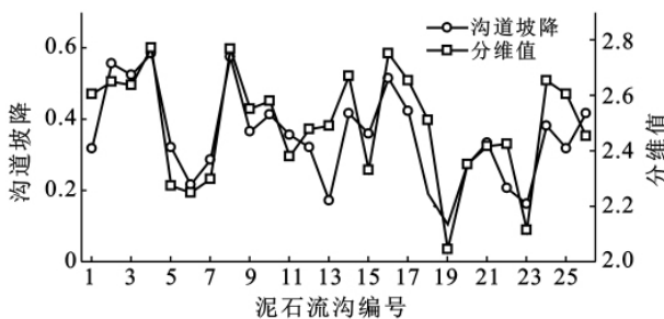
图2 沟道坡降对泥石流堆积物分维值的影响
