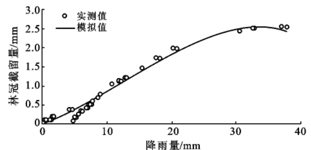
图 1 研究区截留量与林外降雨量的关系
