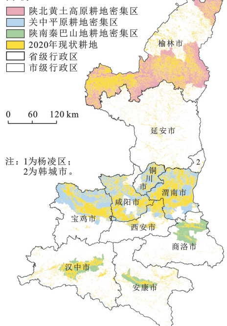
图 2 陕西省耕地密集程度分区
